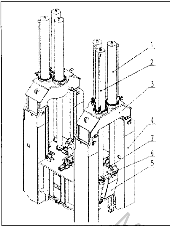
Hình A2.2.2 Cấu tạo của cơ cấu ép cọc: 1, 2 – Các xi lanh thủy lực ép cọc (chính và phụ); 3 – Dầm ngang đỡ các xi lanh thủy lực ép cọc; 4 – Trụ đỡ hướng dẫn ép cọc; 5 - Hộp kẹp cọc; 6 - Ấc và chốt ghép cần của xi lanh thủy lực ép cọc với hộp kẹp cọc; 7 – Bát cầu trên hộp kẹp cọc 5 có nhiệm vụ tiếp nhận đầu dạng cầu tròn của các xi lanh thủy lực ép cọc phụ
