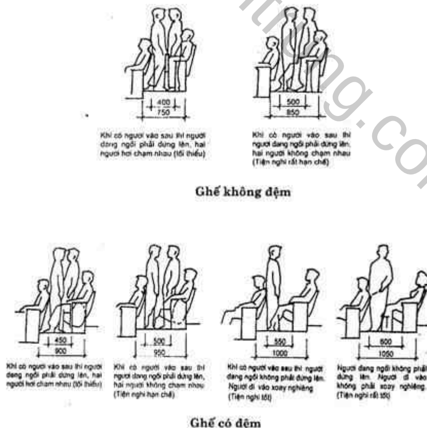
Hình 2: Yêu cầu về khoảng cách giữa các hàng ghế
