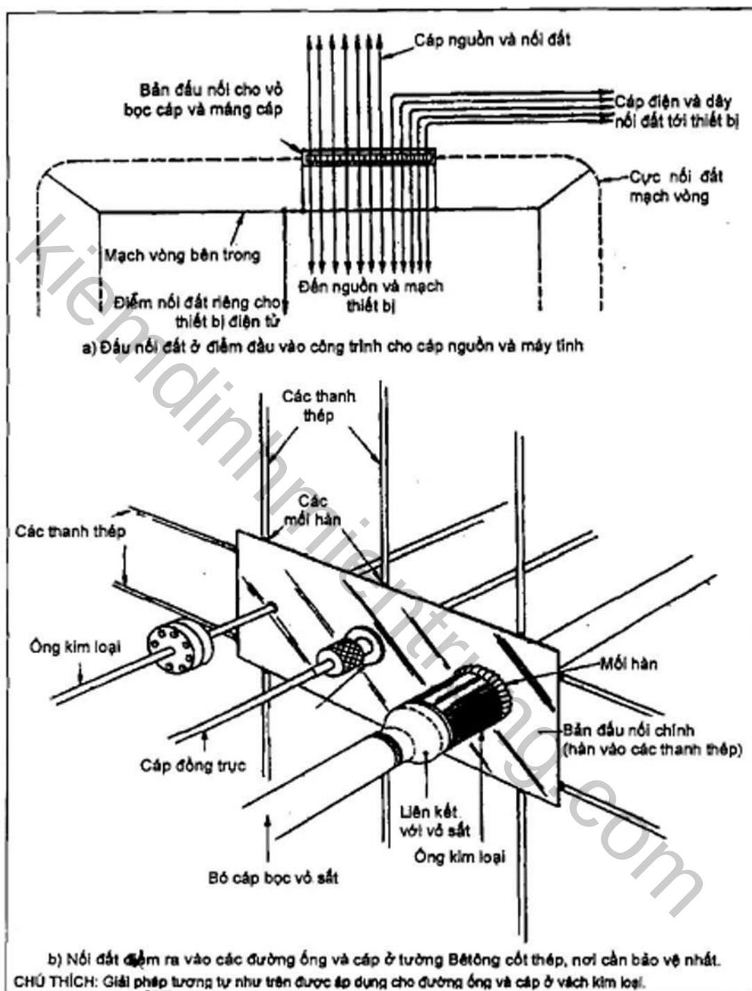
Hình C.7 - Liên kết các đường ống và cáp tại điểm ra vào công trình
