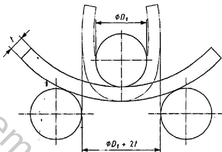
Hình 8 - Minh họa phép thử uốn
