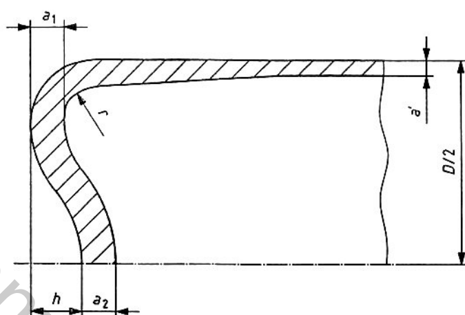
Hình 2 - Đáy lõm chai
