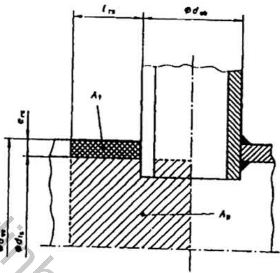
8n) Thân hình trụ với một ống nối được hàn vào với các mối hàn không ngẫu hoàn toàn
