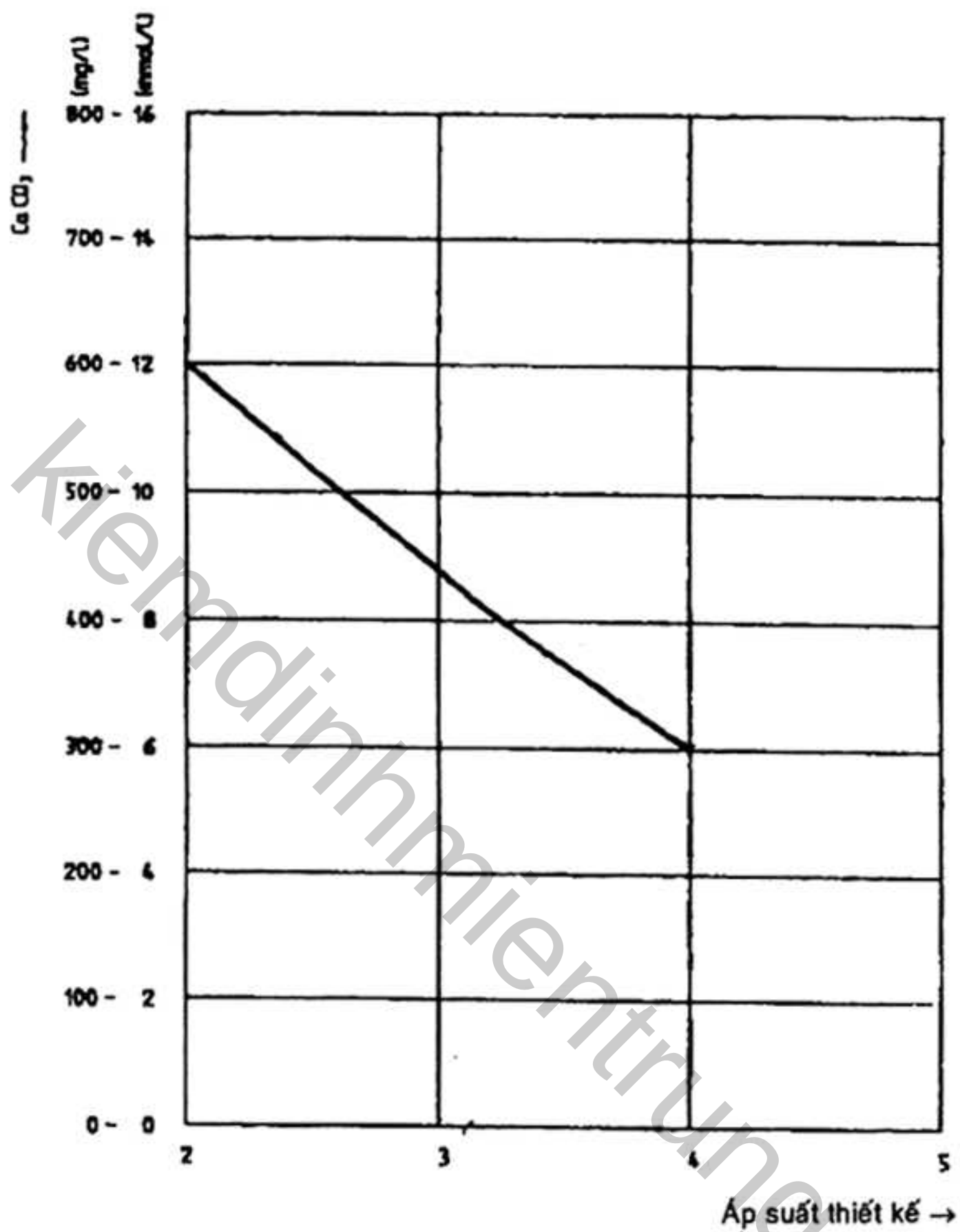
Hình D.2 - Giá trị hướng dẫn đối với độ kiềm ( \text{CaCO}_3 )
