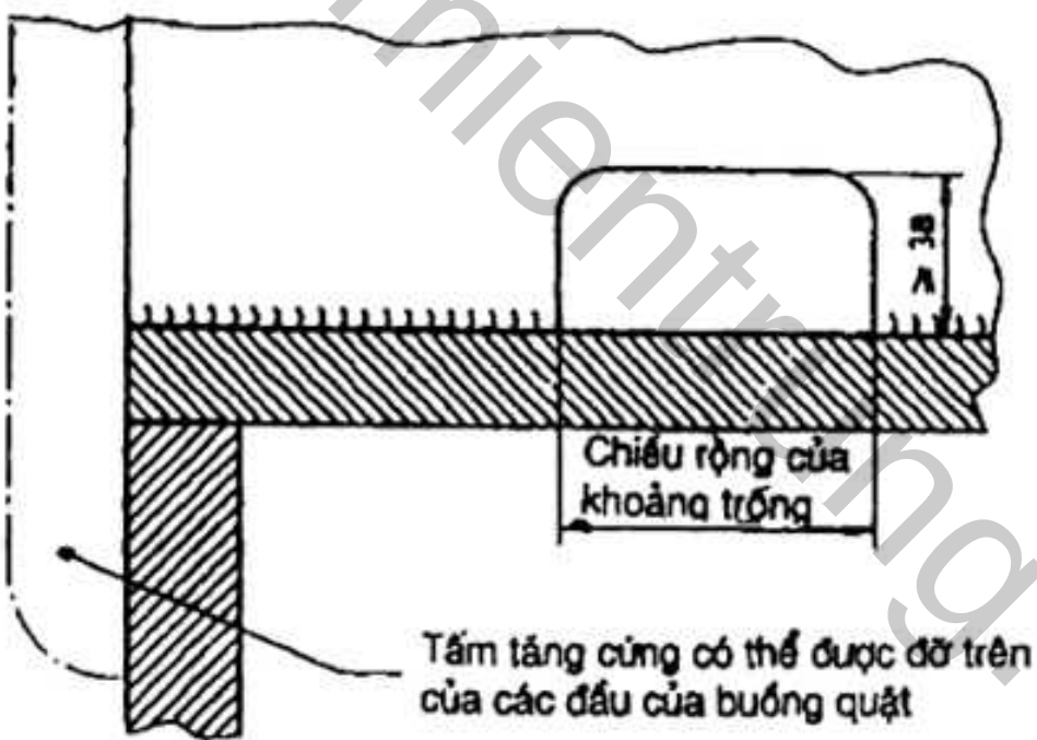
24b) Phương pháp hàn tấm tăng cứng vào buồng quật có các đầu phẳng dẹt
