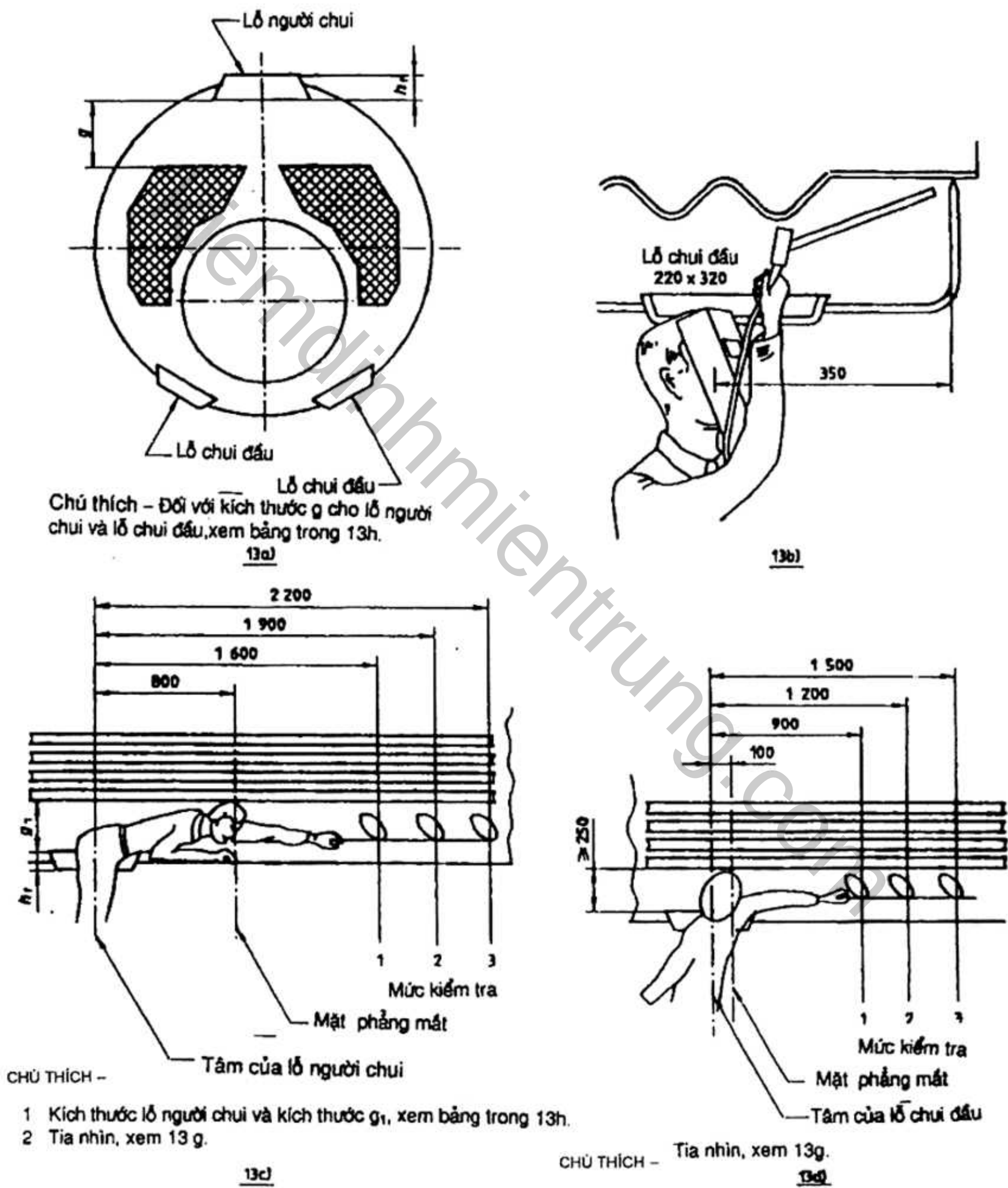
Hình 13 - Lỗ để tiếp cận và kiểm tra
