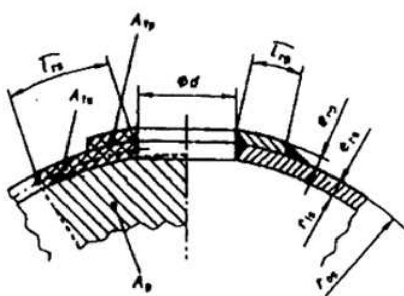
8d) Thân hình cầu và các đáy lồi với các lỗ biệt lập- Gia cường bằng các tấm bù
