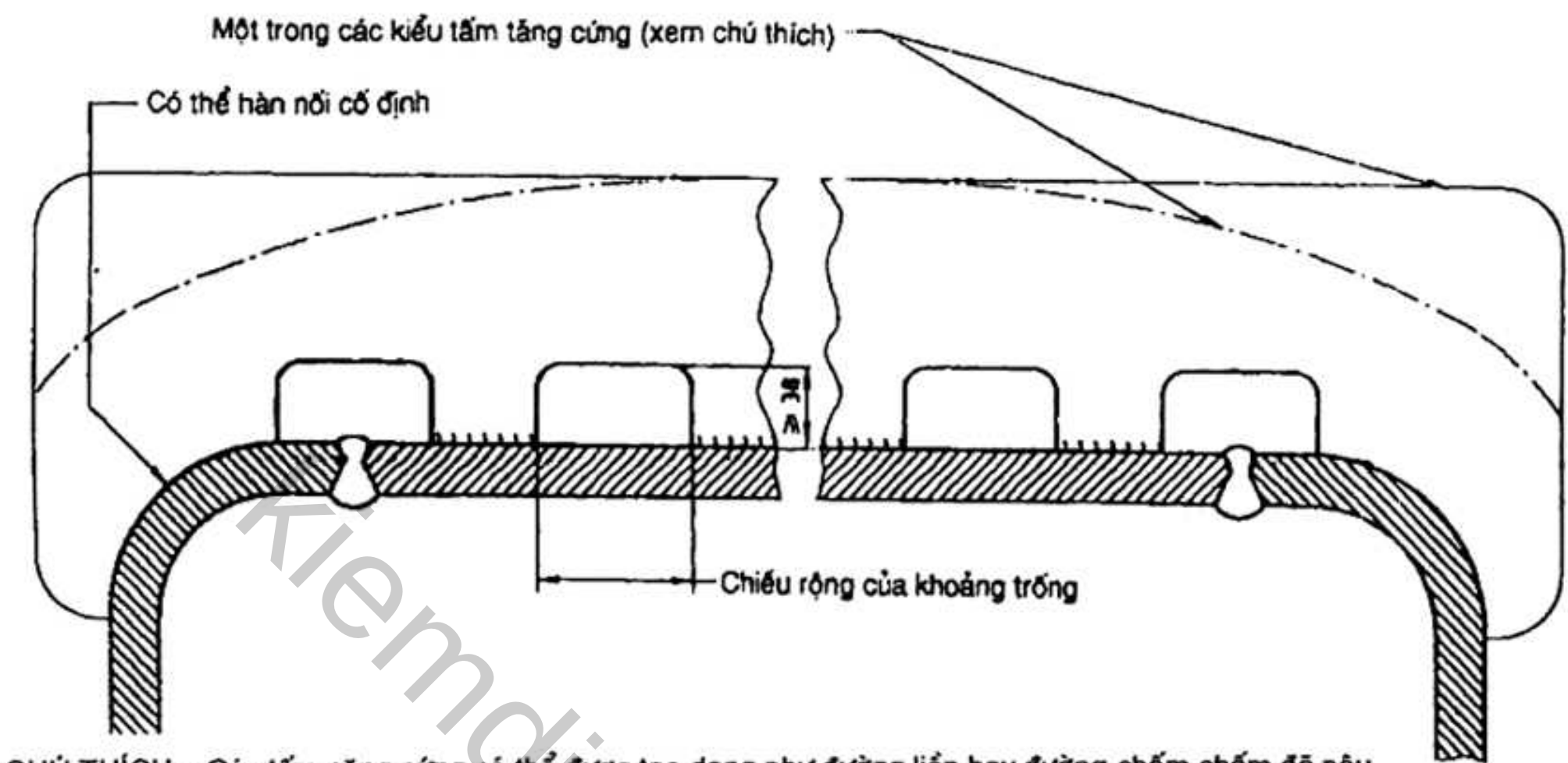
24a) Phương pháp hàn tấm tăng cứng vào buồng quật có gờ mép ở đáy
