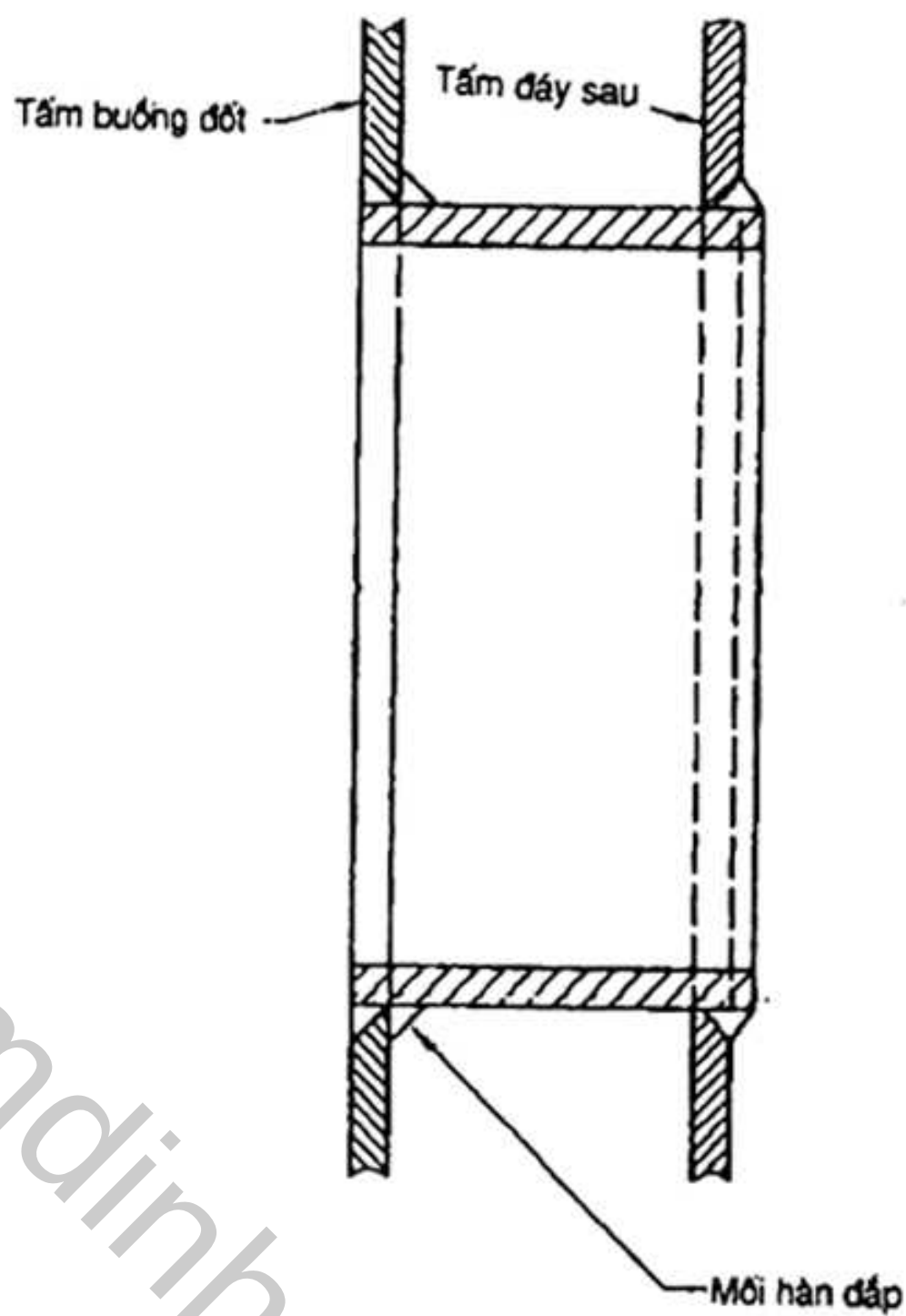
Hình 39 - Lỗ tiệm cận đối với các nổi hơi vách ướ
