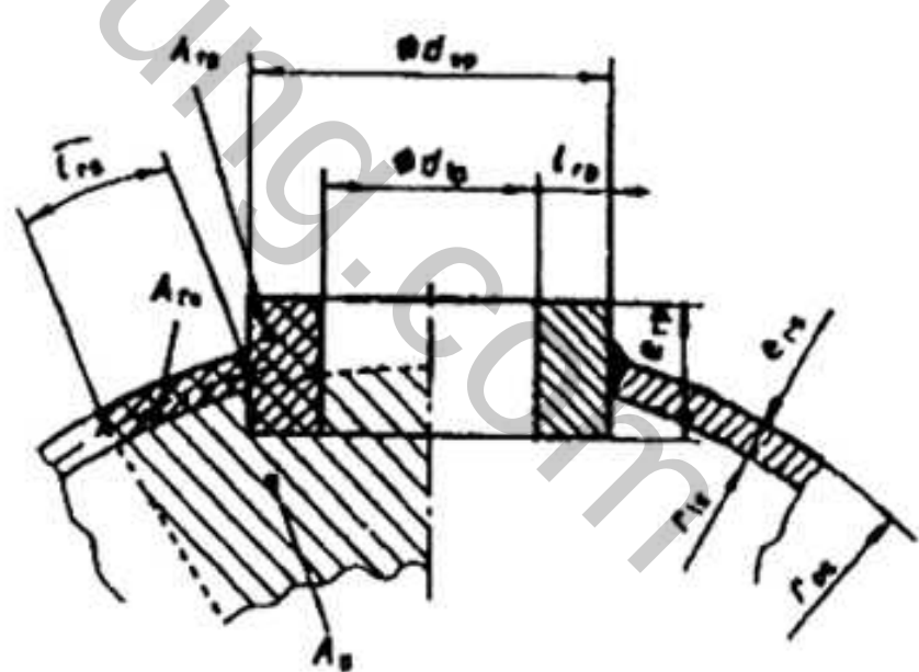
8f) Thân hình cầu và các đáy lồi với các lỗ biệt lập - Gia cường bằng các vòng tăng cứng
