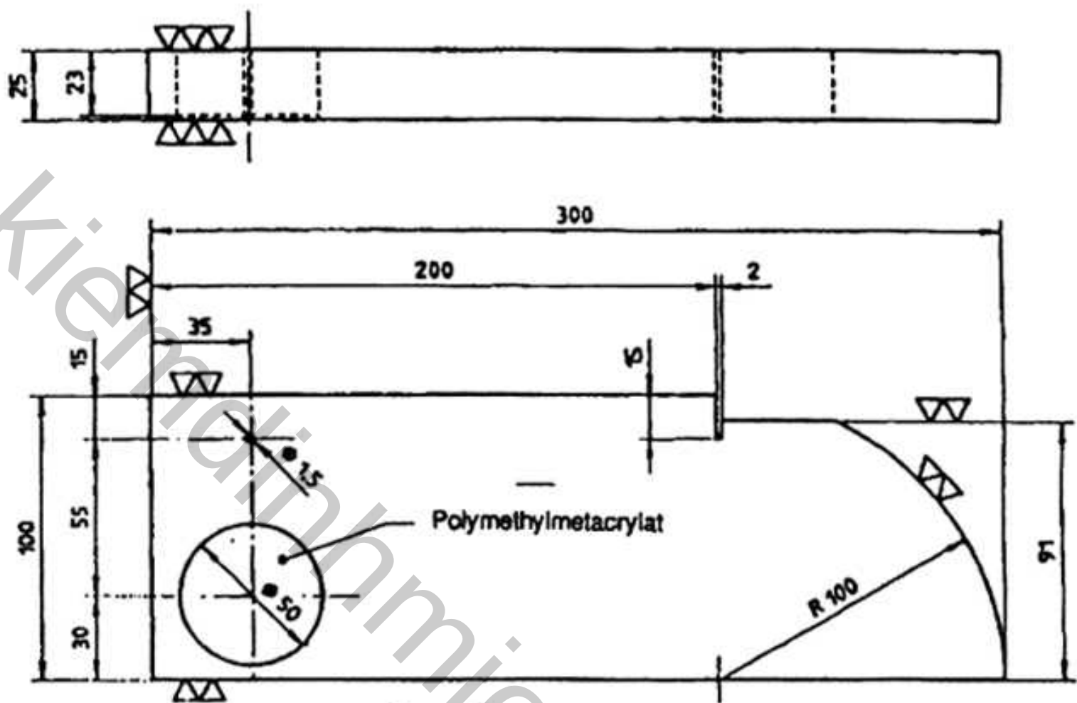
Hình G.1 – Mẫu chuẩn của ISO
