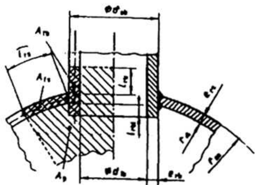
8h) Thân hình cầu và các đáy lồi với các lỗ biệt lập – Gia cường bằng các ống nối
