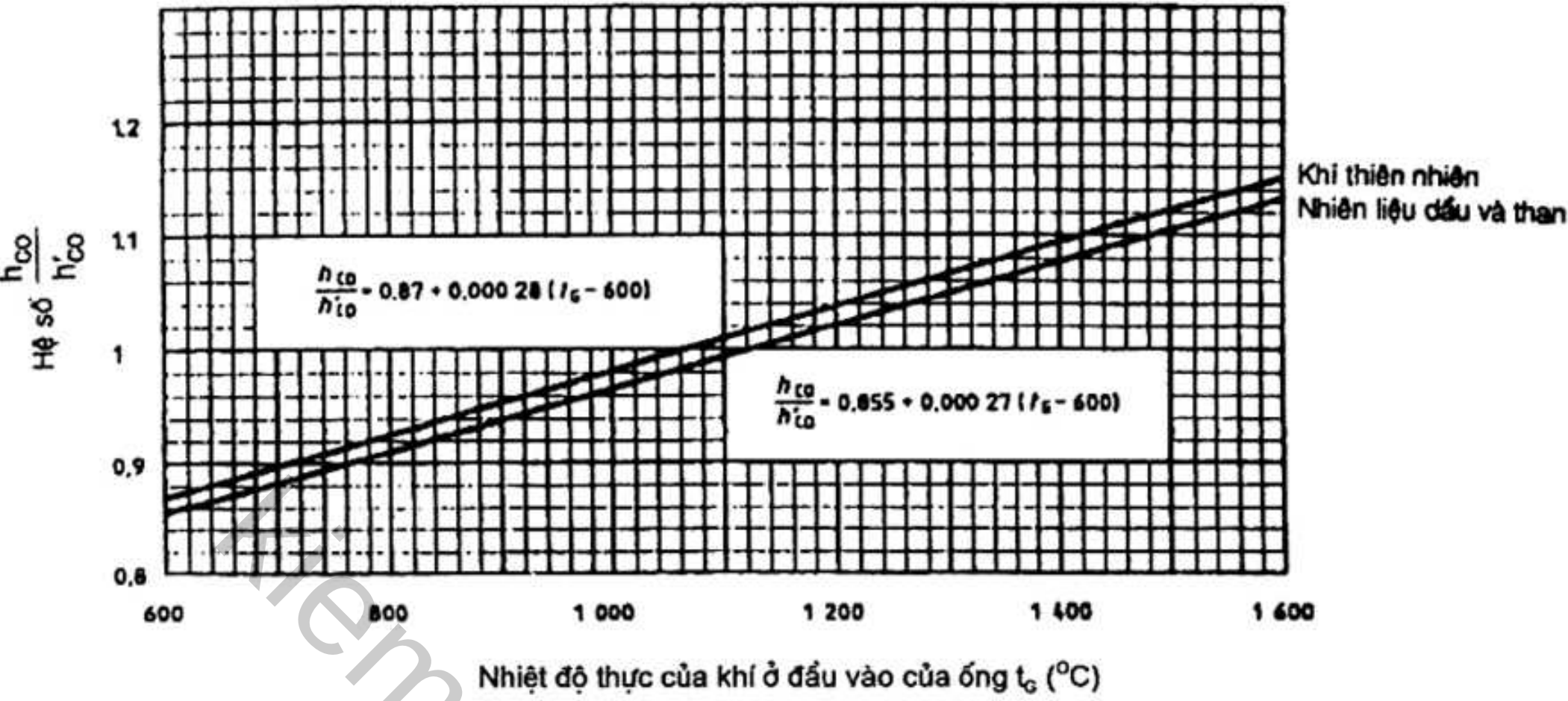
Hình C.5 - Xác định hệ số hiệu chỉnh h_{co}/h'_{co}
