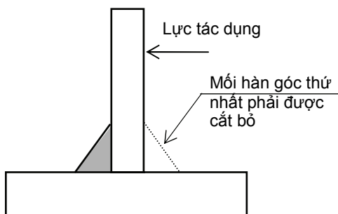
Hình 7. Thử đứt
