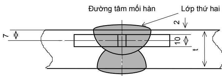
Hình 10. Vị trí của mẫu thử va đập mối hàn giáp mép (đơn vị: mm, t: chiều dày tấm kim loại)
