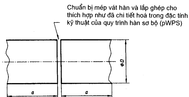
Hình 17. Chi tiết kiểm tra cho mối hàn giáp mép các tấm
