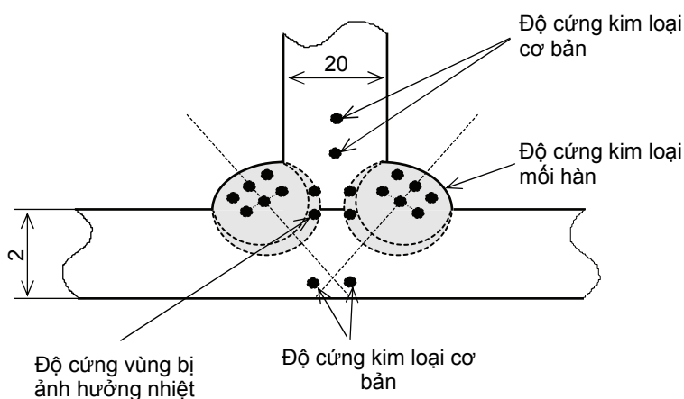
Hình 6. Thử độ cứng (đơn vị: mm)
