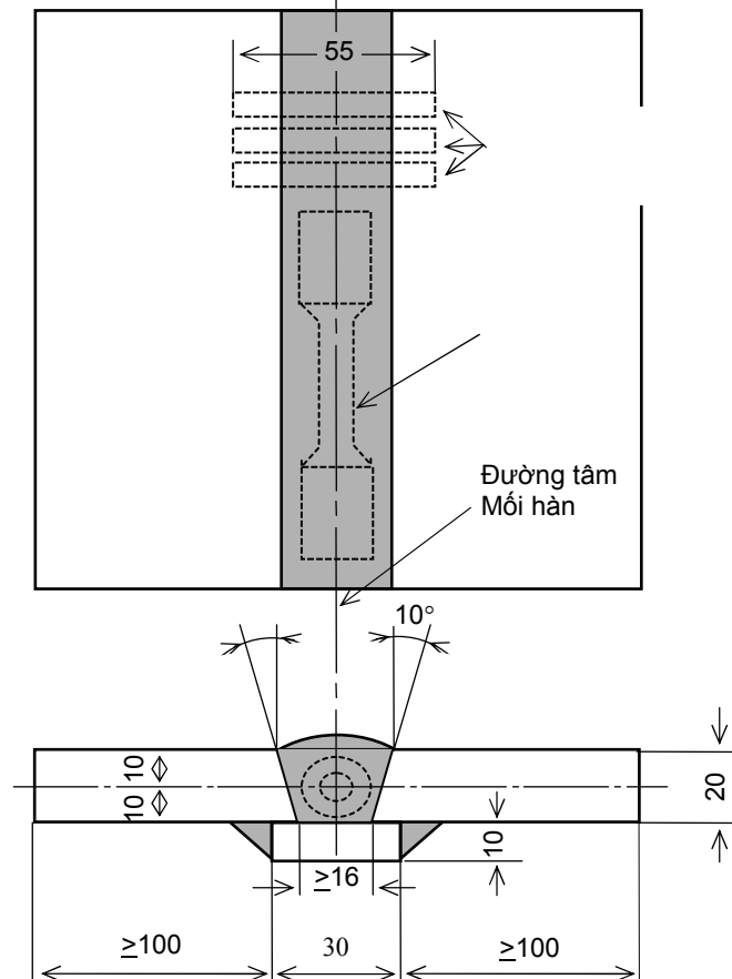
Hình 2. Mẫu thử kim loại dập (đơn vị: mm)
