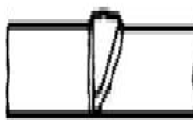
Mối hàn rãnh -J- đơn
