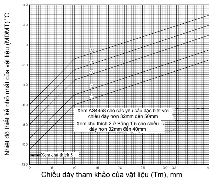
Hình 1 (A). Thép cacbon và cacbon-mangan - Lựa chọn vật liệu khi sử dụng ở nhiệt độ thấp - Hàn không xử lý nhiệt
