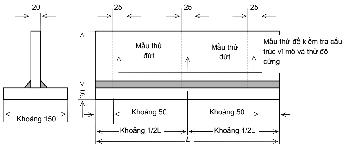
Hình 4. Mẫu thử mối hàn góc (đơn vị: mm)
